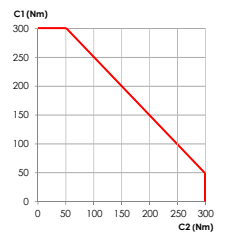
Coppie prelevabili per impiego simultaneo dei 2 utilizzi Max torque for using 2 outputs simultaneously
